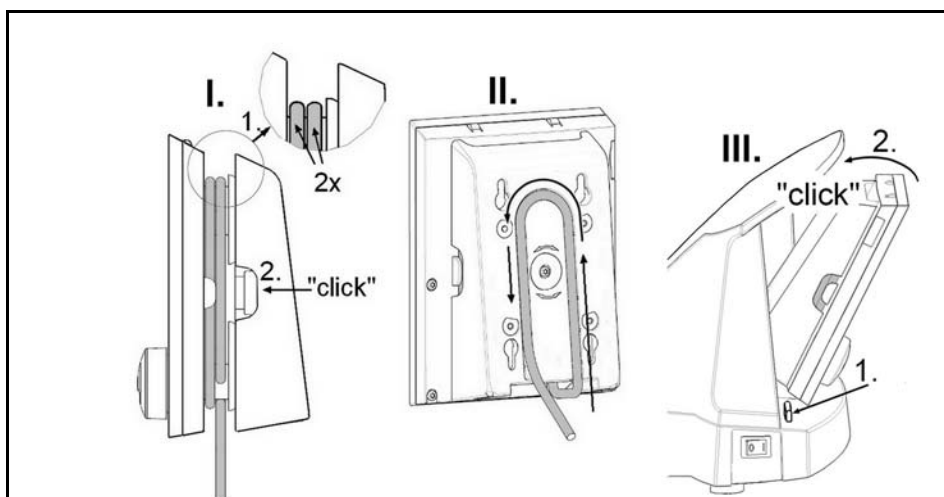
240. Installer le panneau de contrôle sur l'appareil de base
